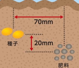
【側条施肥のイメージ】
